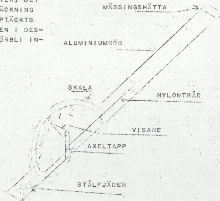
W. B. SMITH'S FÄLTMÄTARE.
